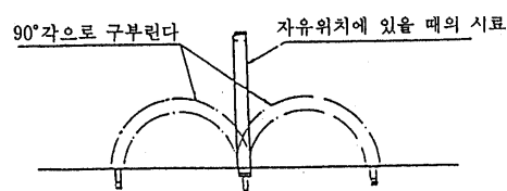
그림 3.8.1.3 호스의 내한성능시험시 굽힘방법
