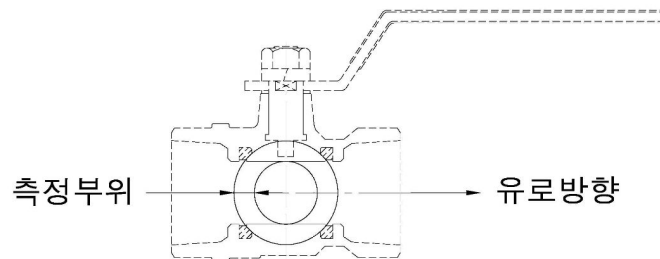
그림 3.3.1 볼 중심부 두께 측정부
