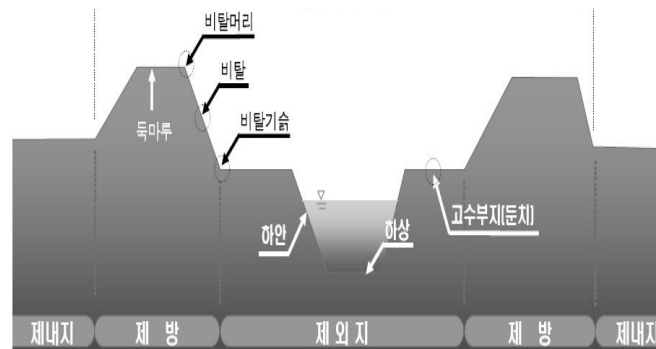
그림 1.3.9 하천구역
