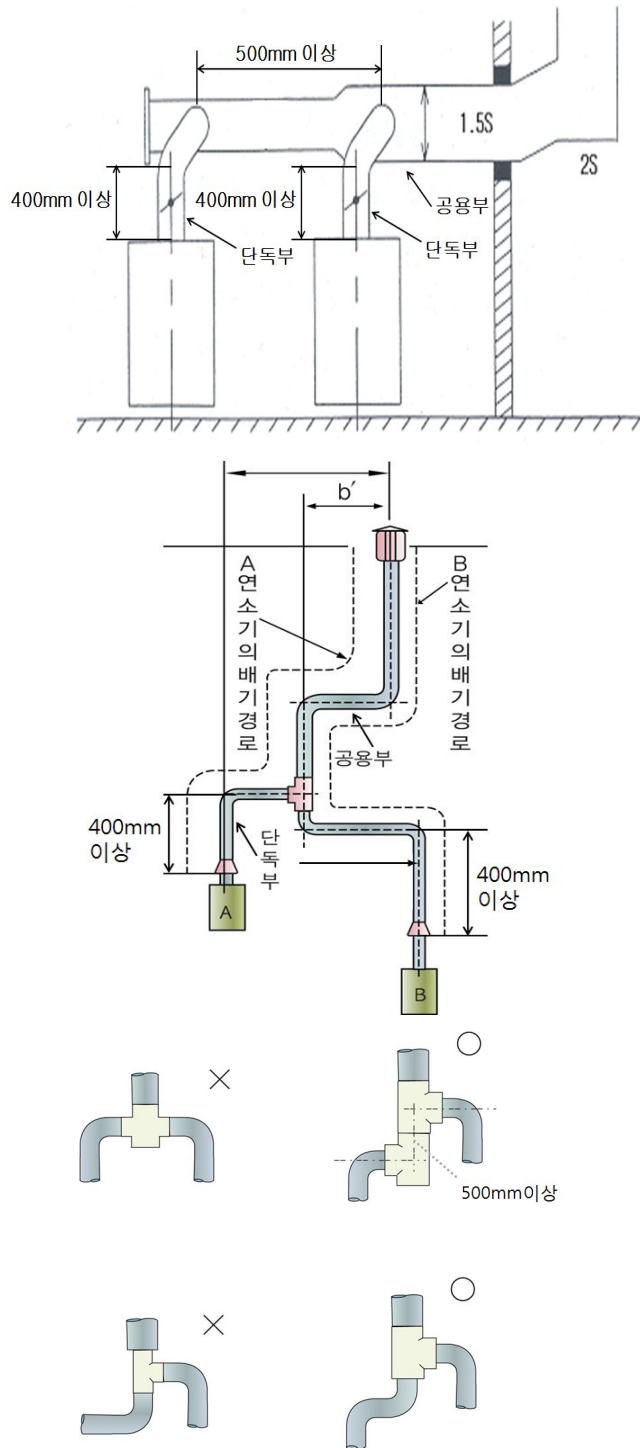
그림 2.7.1.3.2 복합 배기통의 설치 예
