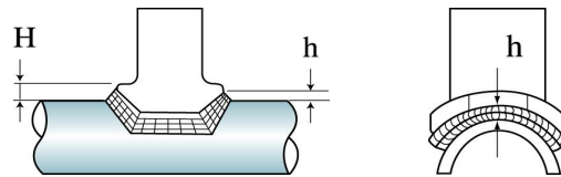
그림 2.5.3.11.7④ 비드의 높이(h) 및 이음관 높이(H)
