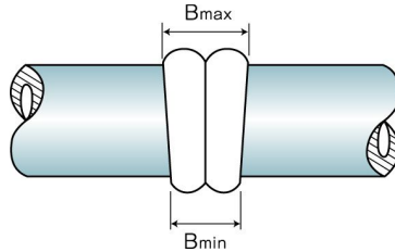
그림 2.5.3.11.7② 비드폭의 최소 및 최대치 예
