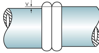
그림 2.5.3.11.7① 이음부의 연결오차(v)
