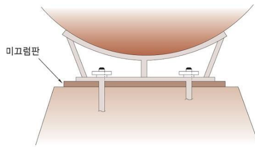
그림 2.2.3.5.3 미끄럼판의 설치방법
