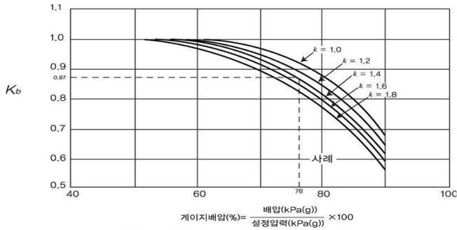
그림 2.8.1.4.1(2) Conventional 안전밸브 배압보정계수
