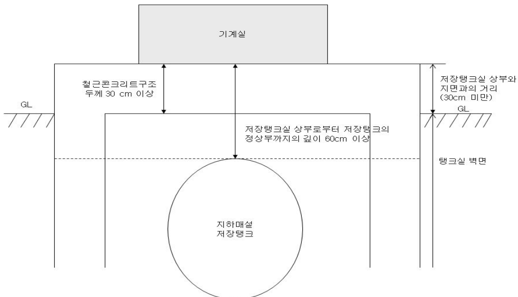
그림 2.3.3.2.5(2) 지하매설 저장탱크 단면도
