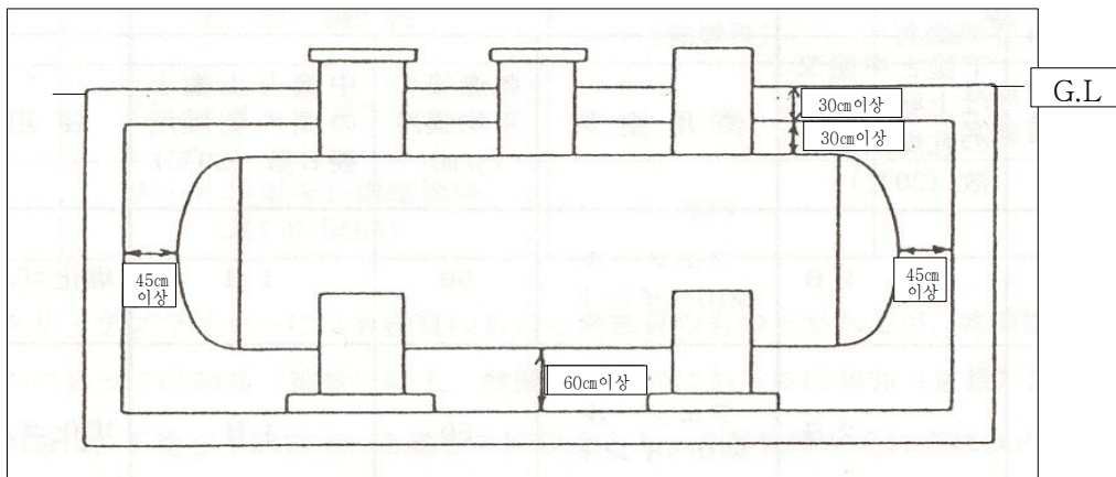
그림 2.3.3.2.5(1) 저장탱크 외면과 저장탱크실 내벽의 이격거리
