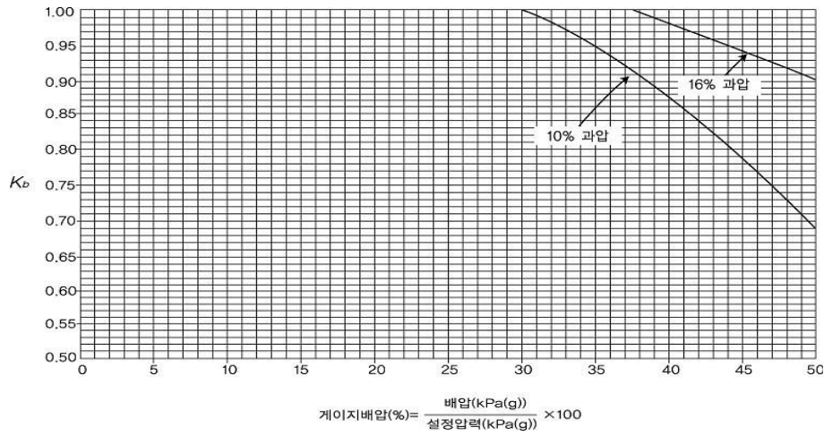
그림 2.8.1.4.1(2) 밸런스 벨로우즈형 안전밸브 배압보정계수
