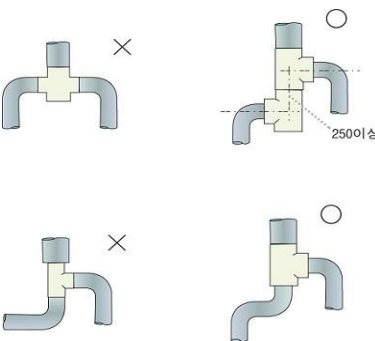
그림 2.7.1.3.1(3) 복합배기통 설치 예
