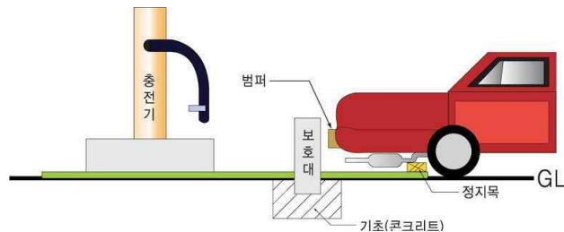
그림 2.3.3.4 보호대 설치방법
