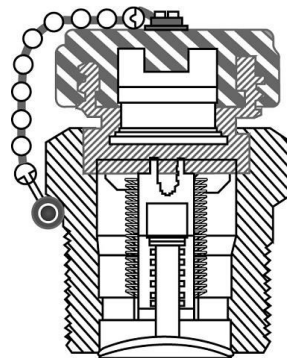
그림 2.3.3.5.1(8)② 세이프티카프링의 암카프링 구조 및 치수의 예(벌크로리용)
