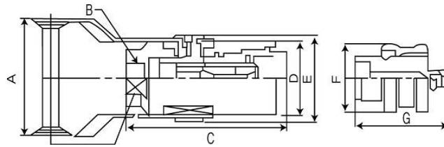
그림 2.3.3.5.1(8)① 세이프티카프링의 슛카프링 구조 및 치수의 예(소형저장탱크용)
