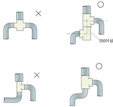
그림 2.7.1.3.1(3) 복합배기통 설치 예
