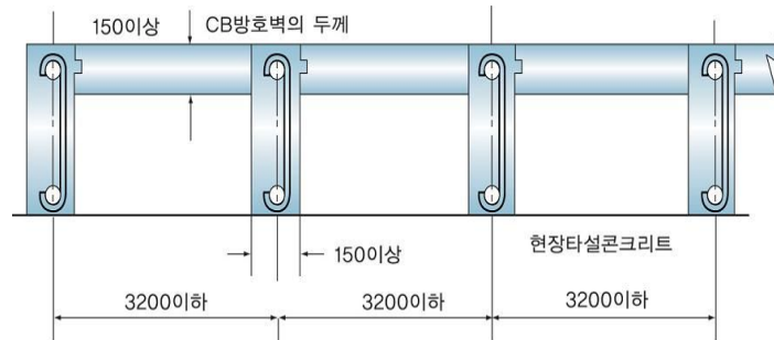
그림 2.9.2.2.2 보조벽의 배치
