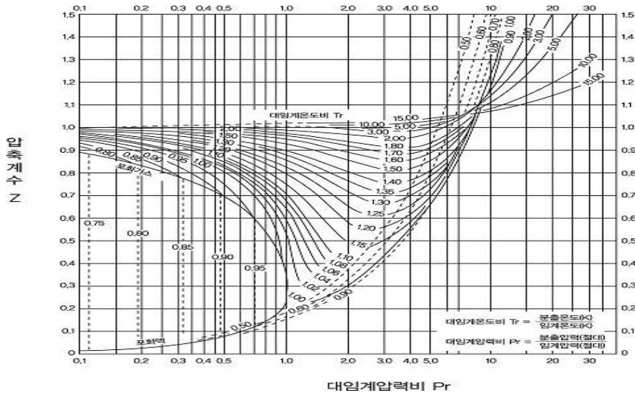
그림 2.8.1.4.1(2)④ 압축계수
