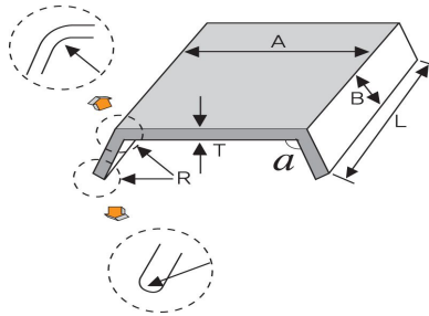
그림 2.5.7.5.3 보호판의 치수
