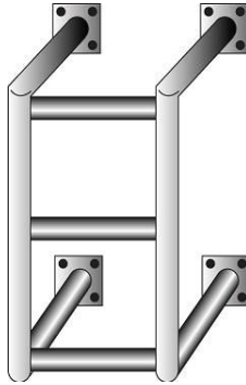
그림 2.5.7.6.9(2)② “ㄱ” 형태로 가공한 강관제 구조물에 의한 방호조치
