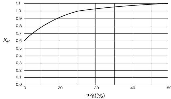
그림 2.8.1.4(2)ⓐ 과압보정계수
