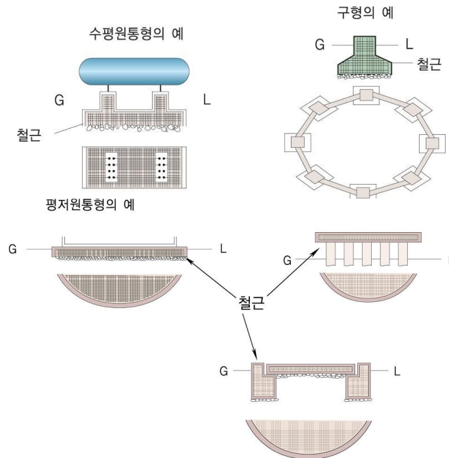
그림 2.2.2.4 저장탱크의 수평기초면
