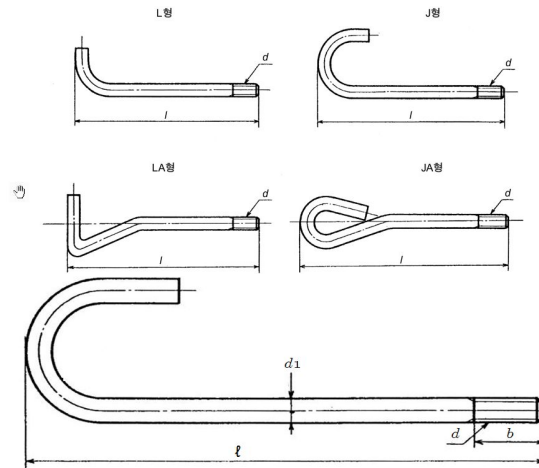
그림 2.2.3.3.1 앵커볼트의 모양
