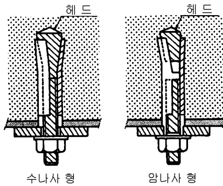
그림 B7.1.2.1.1(2) 금속확장 앵커볼트
