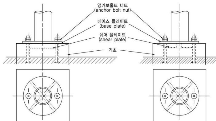
그림 2.2.3.6 구형저장탱크 받침대와 기초에 앵커볼트 체결방법
