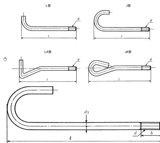
그림 2.2.3.3.1 앵커볼트의 모양
