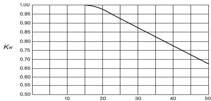
그림 2.7.1.4(2)⑤ 아음속계수
