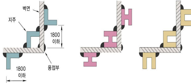
그림 2.8.2.3.4 지주의 설치방법
