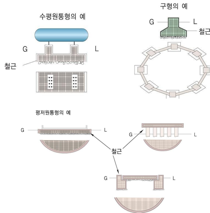
그림 2.2.2.4 저장탱크의 수평기초면
