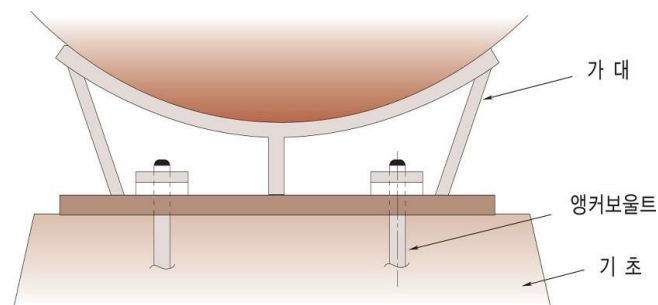
그림 2.2.3.4 앵커보울트의 고정방법
