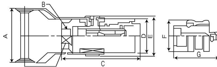
그림 2.3.3.2.4(1)① 세이프티커플링의 스키프링 구조 및 치수의 예시(소형저장탱크용)
