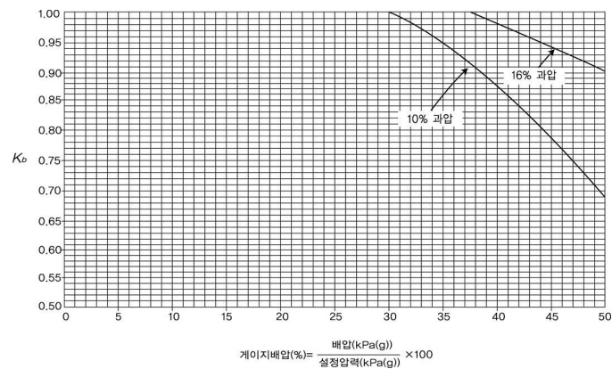
그림 2.6.1.4(2)② 밸런스 벨로우즈형 안전밸브 배압보정계수
