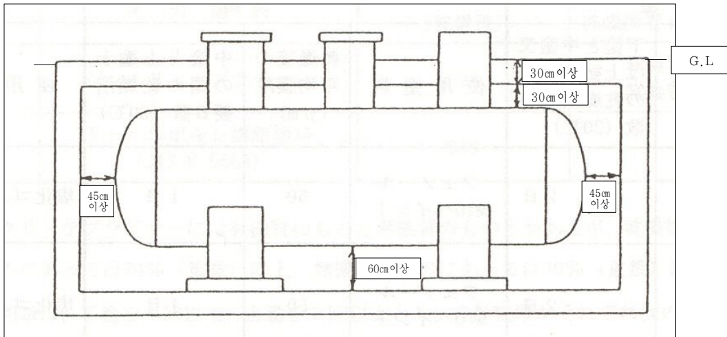
그림 2.3.3.1.2(5-1) 저장탱크 외면과 저장탱크실 내벽의 이격거리
