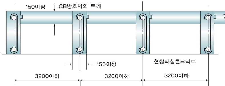
그림 2.7.2.2.2 보조벽의 배치
