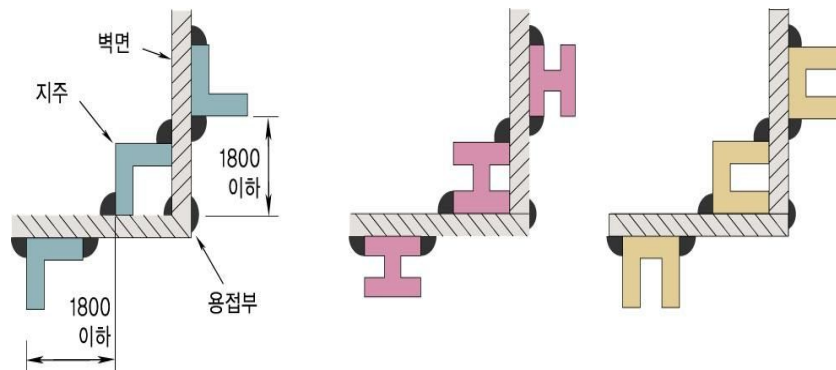
그림 2.7.2.3.4 지주의 설치방법
