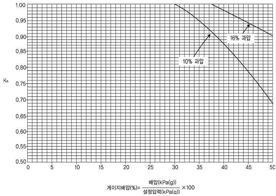
그림 2.6.1.4
