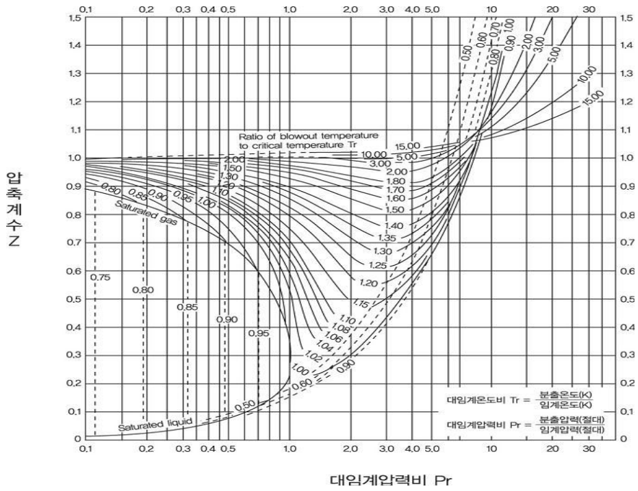
그림 2.6.1.4④ 압축계수
