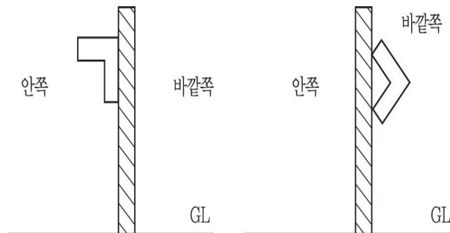
그림 2.7.2.3.2 강판제 방호벽의 앵글강 보강
