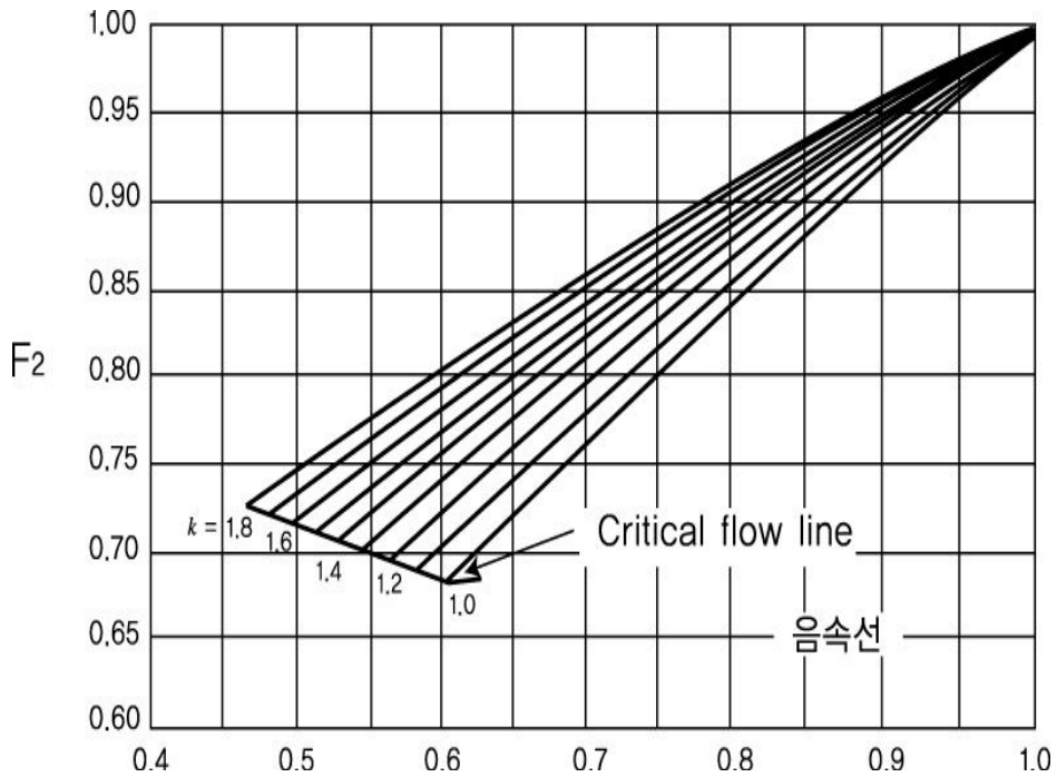
그림 2.6.1.4⑤ 아음속계수
