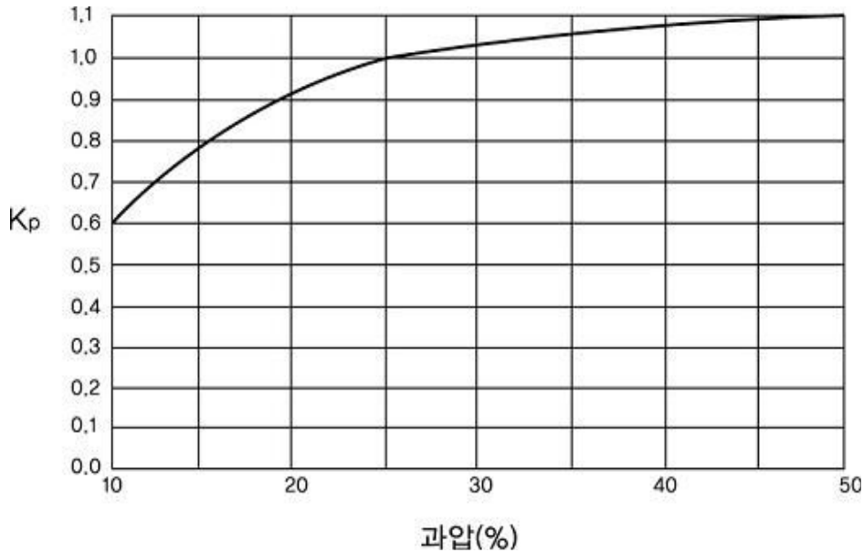
그림 2.6.1.4⑧ 과압보정계수
