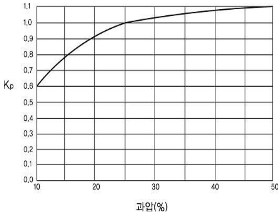
그림 2.6.1.4⑧ 과압보정계수
