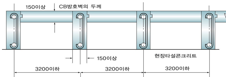
그림 2.7.2.2.2 보조벽의 배치
