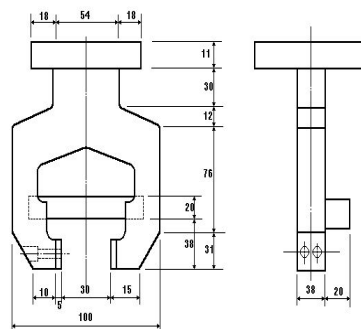
그림 3.11.3 밸브 부착 치구(예시)
