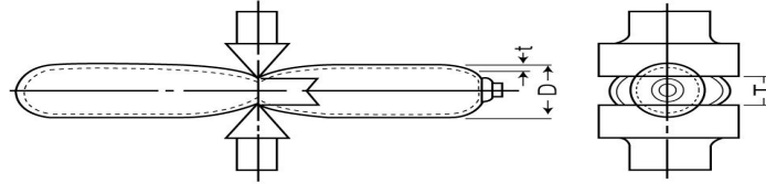
그림 4.4.2.2.1(2)③ 압괴시험용 강제짜기
