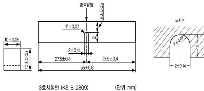
그림 4.4.2.2.1(2)② 제3호 시험편(KS B 0809)
