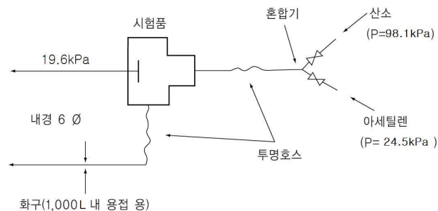
그림 3.8.1.4 역화방지사험 방법
