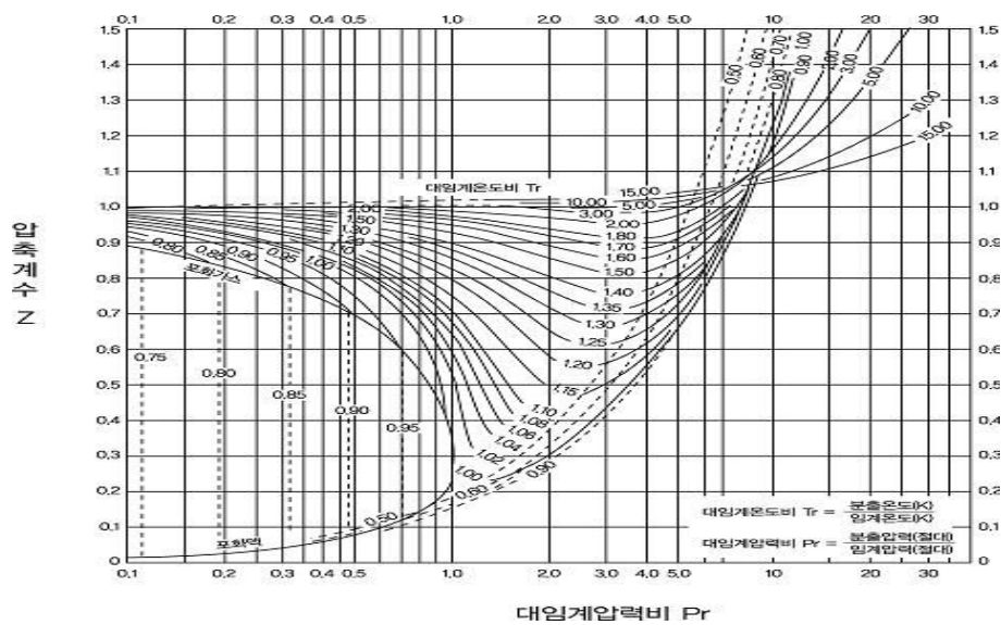
그림 2.8.1.4.1(2)④ 압축계수
