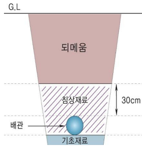
그림 2.5.7.5.5(1) 배관의 매설방법
