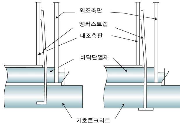
그림 2.2.3.7 평저형 저장탱크의 앵커스트립 설치방법
