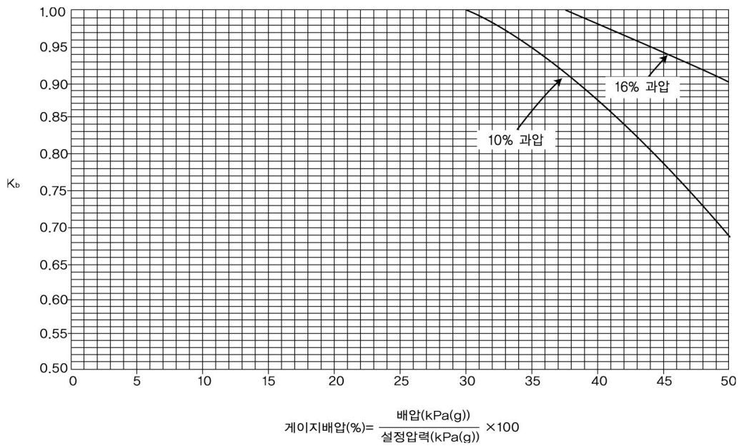
그림 2.6.1.4② 밸런스 벨로우즈형 안전밸브 배압보정계수
