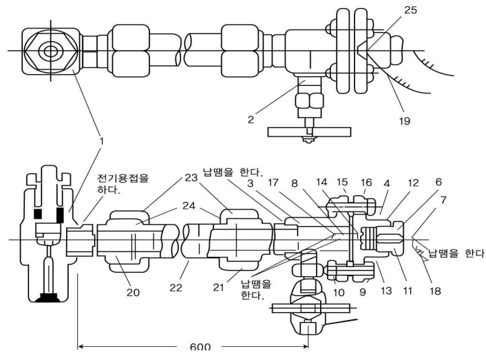
4.4.2.2.1(2)⑱ 역화시험장치
