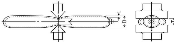
그림 4.4.2.2.1④ 썸기 모양
