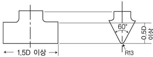
그림 4.4.2.2.1④ 썸기 모양
