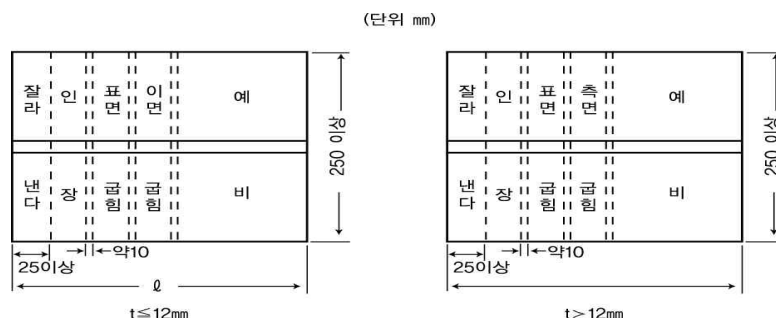
그림 4.4.2.2.1⑩ 시험판
