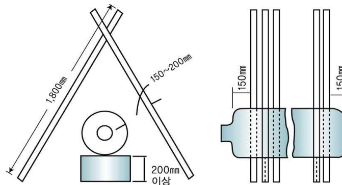
그림 4.4.2.2.1(2)⑯ 주위가열시험
