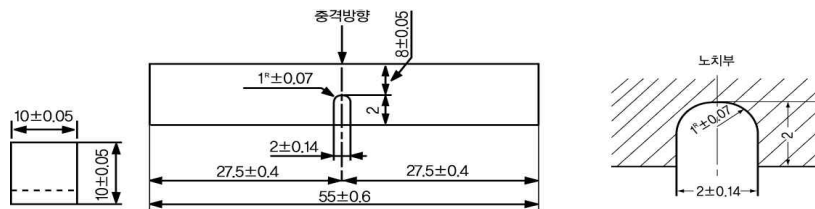
3호시험편 (KS B 0809)
