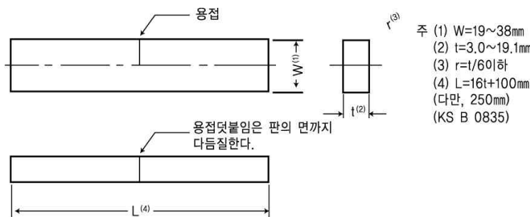
그림 4.4.2.2.1⑫ 맞대기 용접이음의 로울러 굽힘시험의 시험편
