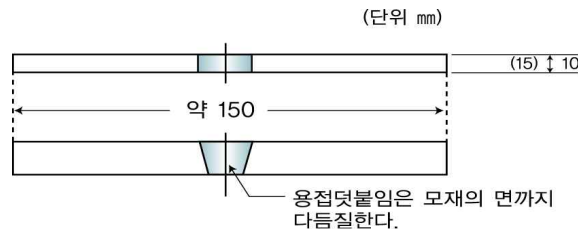
그림 4.4.2.2.1⑭ 측면굽힘 시험편
