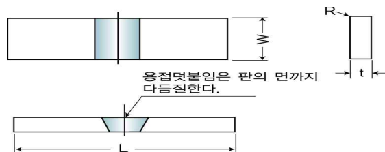
그림 4.4.2.2.1⑫ 맞대기 용접이음의 로울러 굽힘시험의 시험편
