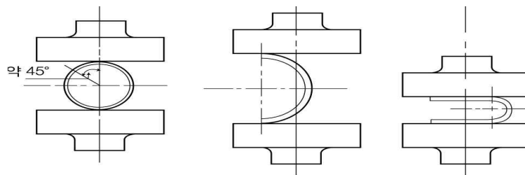
그림 4.4.2.2.1⑥ 중앙부에 길이이음매가 있는 시료의 위치
