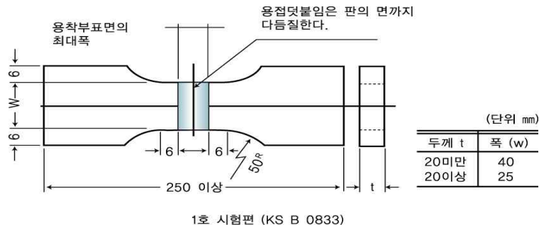
그림 4.4.2.2.1⑩ KS B 0833(맞대기 용접이음의 인장시험방법)의 1호 시험편
