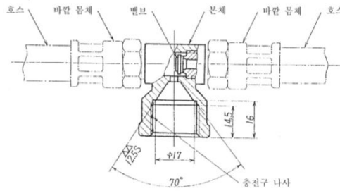
그림 3.4.8 트윈호스의 조정기 연결부 구조
