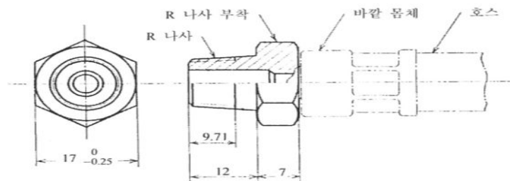
그림 3.4.6 집합관에 연결하는 측도관 이음쇠의 구조 <신설 10.8.31>
