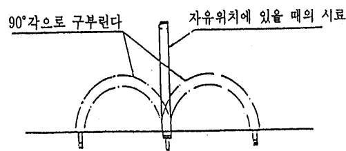
그림 3.8.1.3 호스의 내한성능 시험 <신설 10.8.31>
