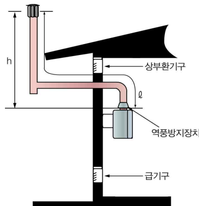
그림 2.7.1.3.1①배기통의 높이
