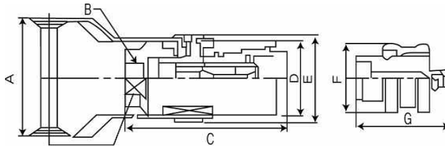
그림 2.3.3.5.1(8)① 세이프터카프링의 스텀카프링 구조 및 치수의 예(소형저장탱크용)
