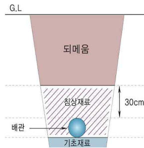
그림 2.5.7.5.5(1) 배관의 매설방법
