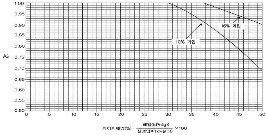
그림 2.8.1.4.1(2) 밸런스 벨로우즈형 안전밸브 배압보정계수
