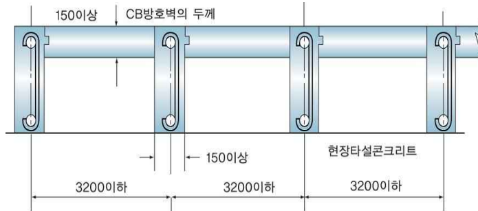
그림 2.9.2.2.2 보조벽의 배치
