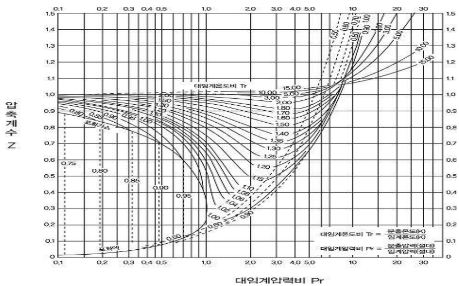
그림 2.8.1.4.1(2) 압축계수
