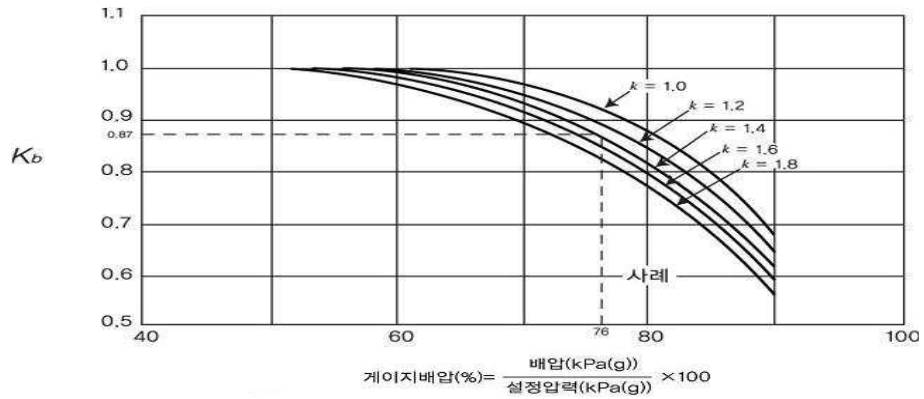
그림 2.8.1.4.1(2) Conventional 안전밸브 배압보정계수
