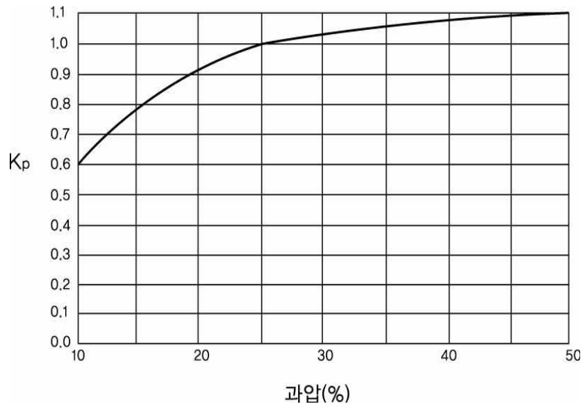
그림 2.8.1.4.2③ 과압보정계수
