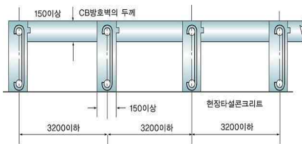
그림 2.9.2.2.2 보조벽의 배치
