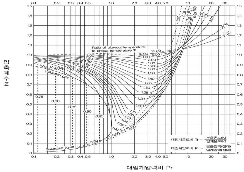
그림 2.8.1.4.1④ 압축계수
