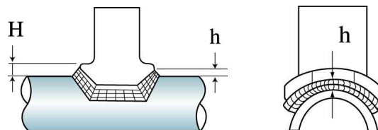
그림 2.5.5.8.7(1)④ 비드의 높이(h) 및 이음관 높이(H)
