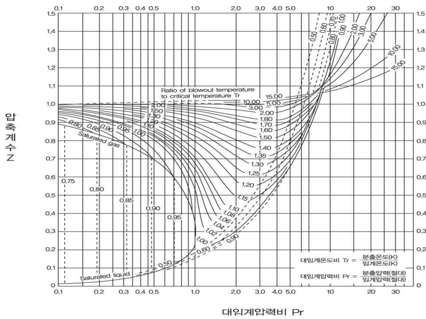
그림 2.7.1.2④ 압축계수
