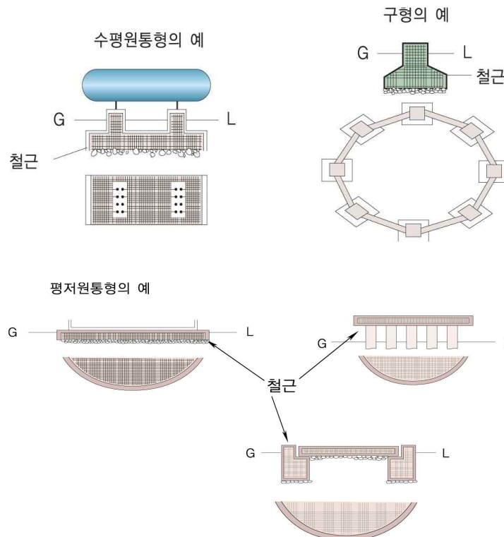
그림 2.2.2.3 저장탱크의 수평기초면
