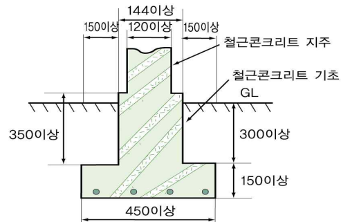
그림 2.8.2.1 철근콘크리트 방호벽의 설치 예
