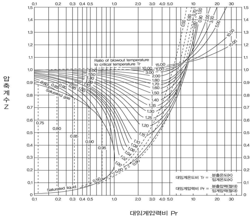
그림 2.7.1.4.1④ 압축계수
