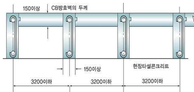
그림 2.8.2.2.2 보조벽의 배치
