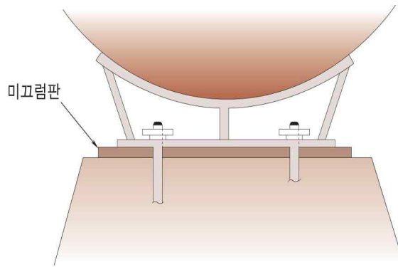
그림 2.2.3.5 미끄럼판의 설치방법
