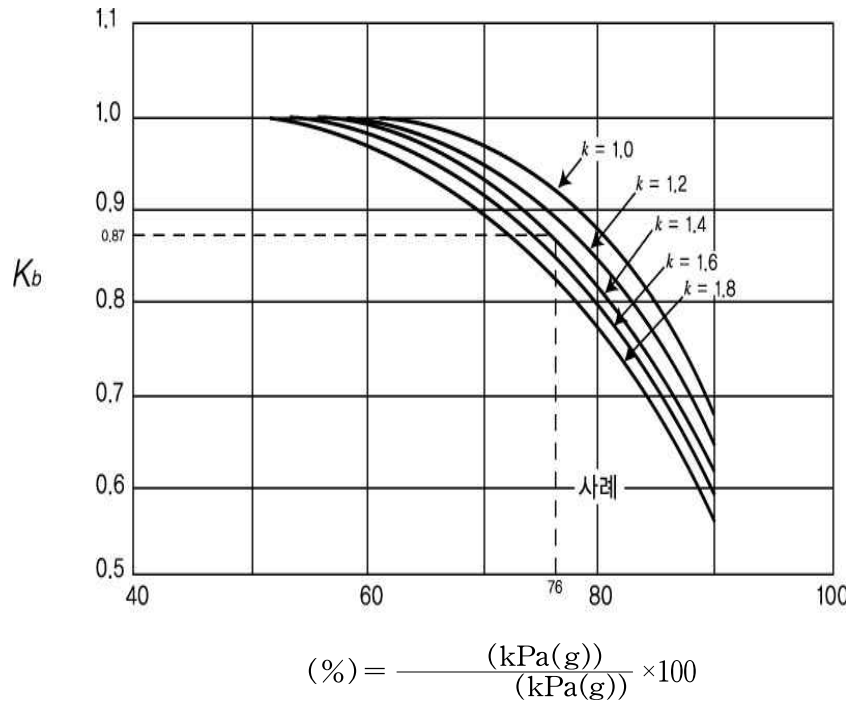
그림 2.7.1.4.1③ Conventional 안전밸브 배압조정계수
