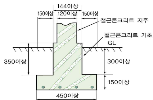
그림 2.8.2.1.2 철근콘크리트 방호벽의 설치 예
