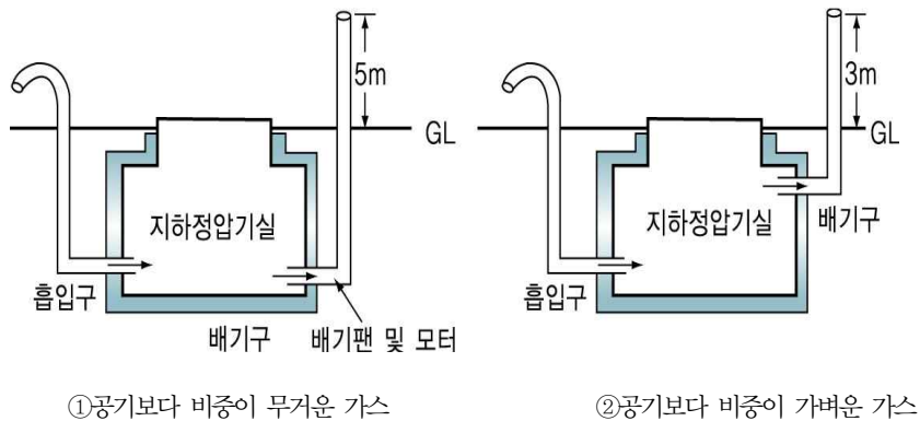
그림 2.6.9.1.3 지하 가스공급시설의 환기구설치
