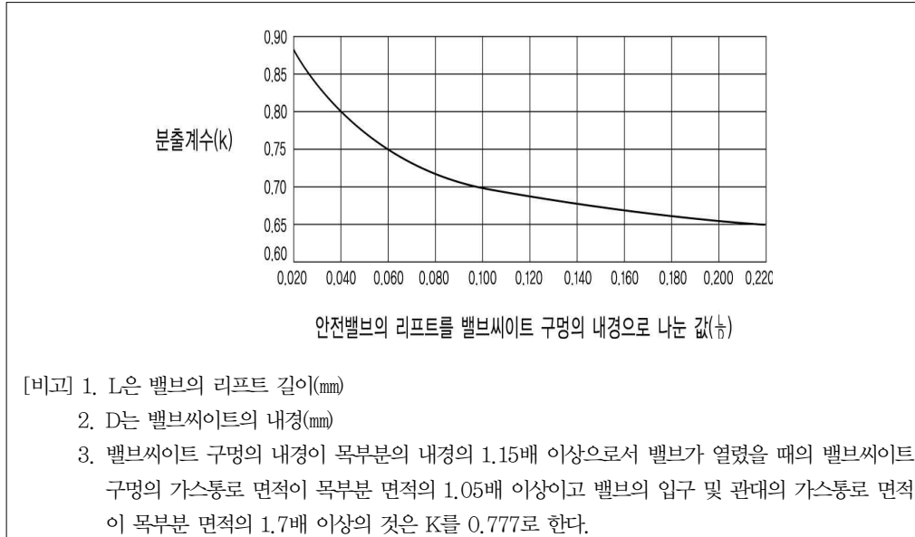
그림 2.6.1.1.2 분출계수
