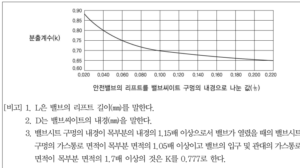
그림 2.6.1.1.4 분출계수
