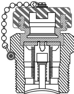
그림 2.3.3.2.4(1)② 세이프티커플링의 암커플링 구조 및 치수의 예시(벌크로리용)
