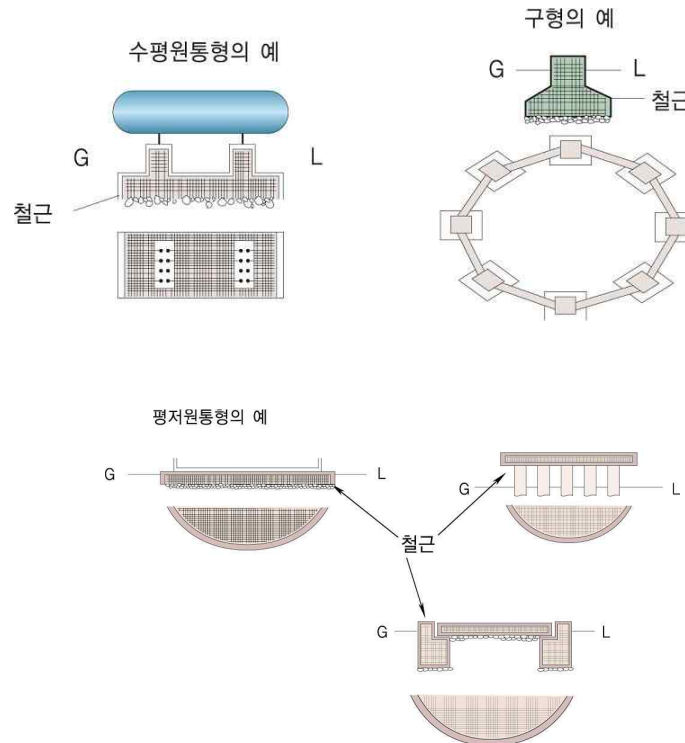
그림 2.2.2.4 저장탱크의 수평기초면
