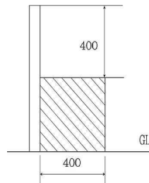
그림 2.7.2.2.3 보조벽의 높이
