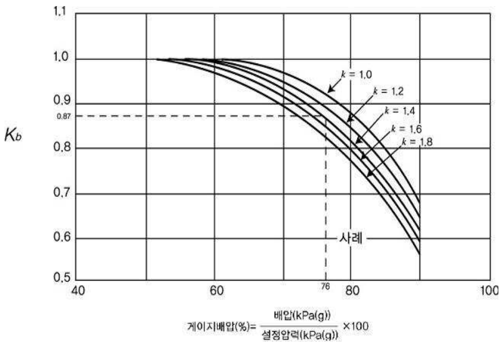
그림 2.6.1.4③ Conventional 안전밸브 배압조정계수
