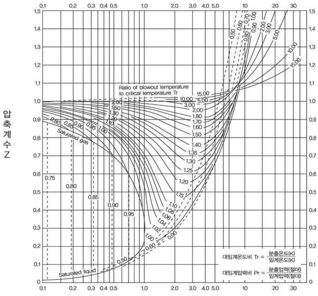
대임계압력비 Pr
