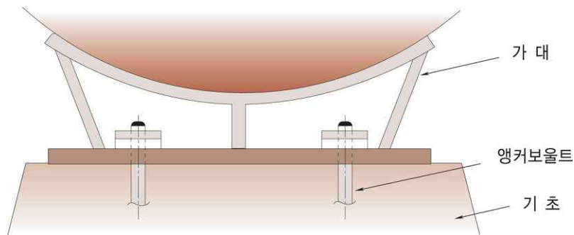
그림 2.2.3.4 앵커보울트의 고정방법
