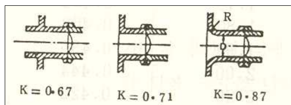
그림 A3.2(1)② 파열관의 분출계수
