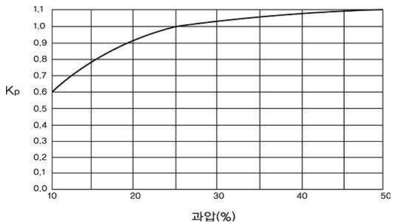
그림 2.6.1.4⑧ 과압보정계수
