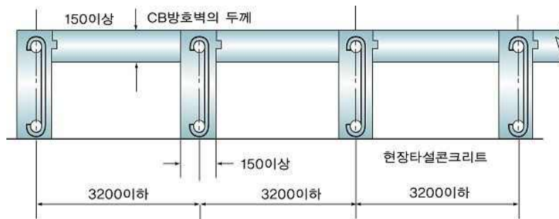
그림 2.7.2.2.2 보조벽의 배치
