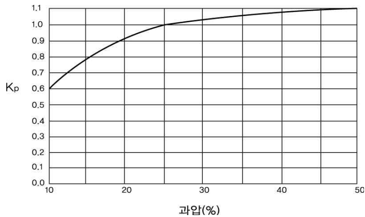
그림 3.4.6.3.1⑧ 과압보정계수
