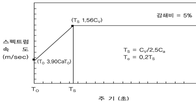
그림 2.4.6.1.1 표준설계응답스펙트럼
