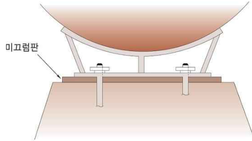
그림 2.2.3.5.3 미끄럼판의 설치방법
