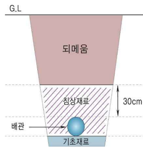
그림 2.5.7.5.1(5) 배관의 매설방법
