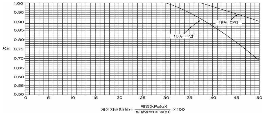
그림 2.8.1.4.1(2)② 밸런스 밸로우즈형 안전밸브 배압보정계수
