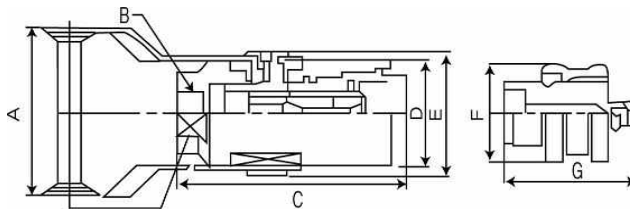
그림 2.3.3.5.1(8)① 세이프터카프링의 슛카프링 구조 및 치수의 예(소형저장탱크용)
