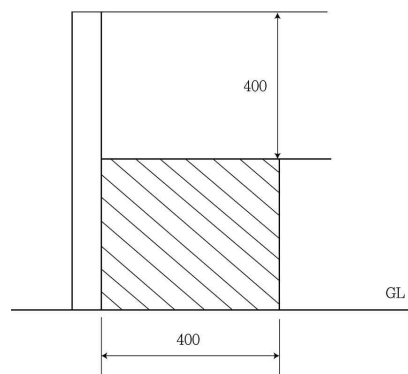
그림 2.9.2.2.3 보조벽의 높이
