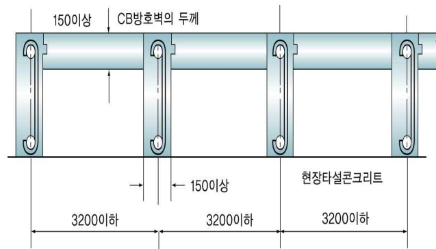
그림 2.9.2.2.2 보조벽의 배치
