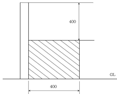
그림 2.9.2.2.3 보조벽의 높이
