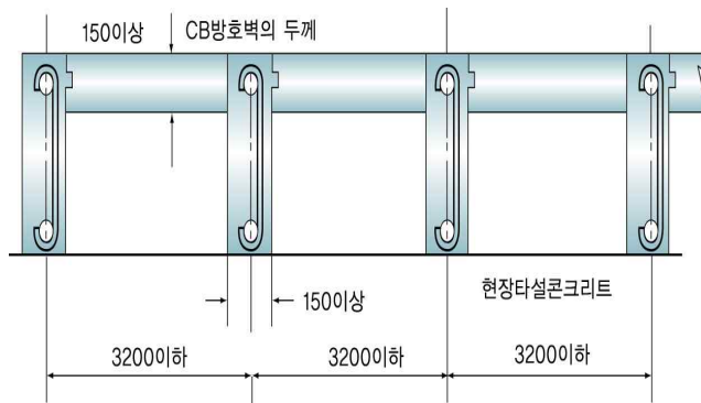
그림 2.9.2.2.2 보조벽의 배치
