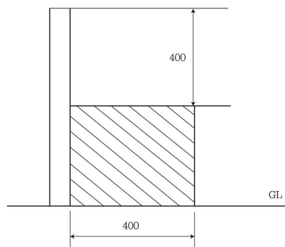
그림 2.8.2.2.3 보조벽의 높이
