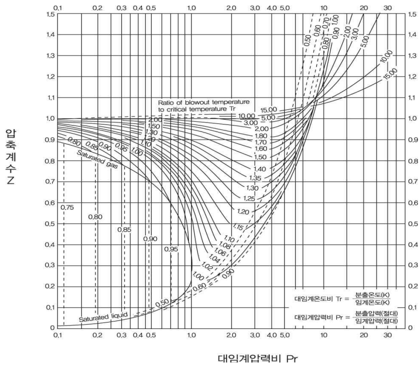
그림 2.7.1.4.1④ 압축계수
