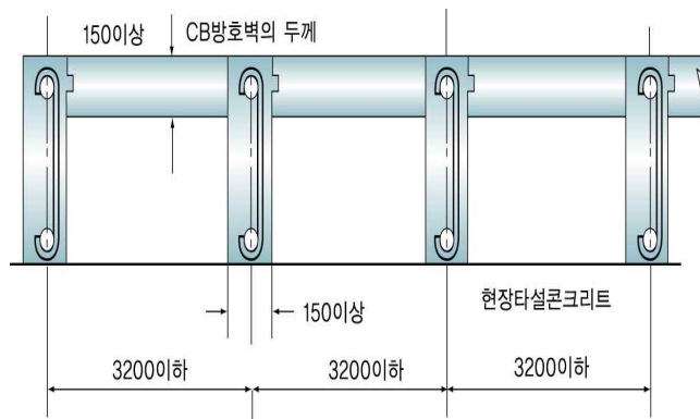
그림 2.8.2.2.2 보조벽의 배치
