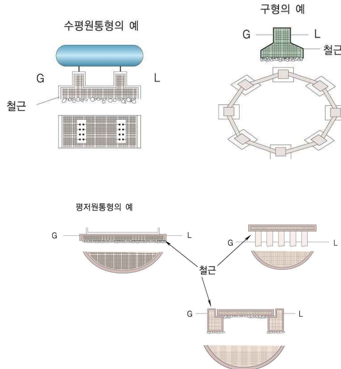
그림 2.2.2.4 저장탱크의 수평기초면
