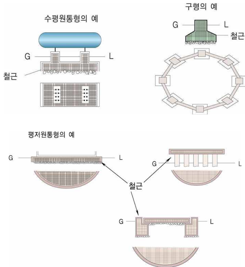
그림 2.2.2.3 저장탱크의 수평기초면
