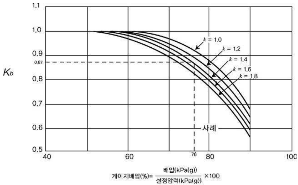
그림 2.6.1.4③ Conventional 안전밸브 배압조정계수
