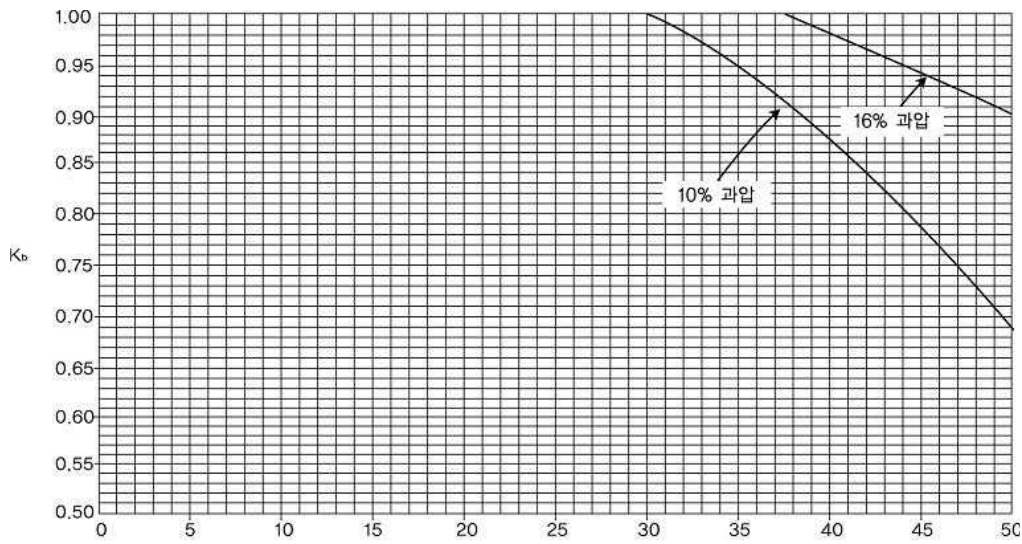
그림 2.6.1.4② 밸런스 벨로우즈형 안전밸브 배압보정계수
