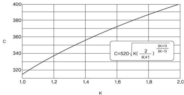
그림 2.6.1.4① 열용량비 k=C_p/C_v
