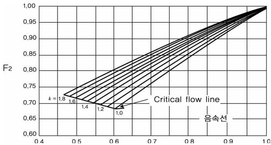
그림 2.6.1.4⑤ 아음속계수
