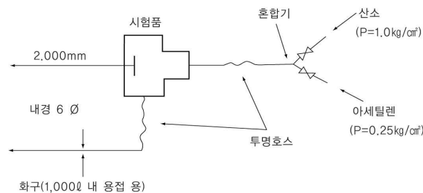
그림 3.8.1.4 역화방지시험 방법
